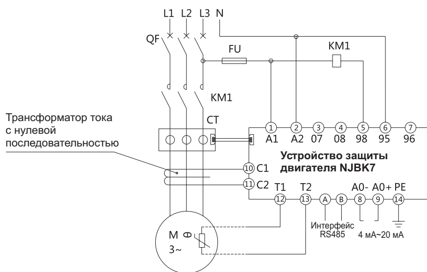
Рис. 10. Схема соединений, прямой запуск
