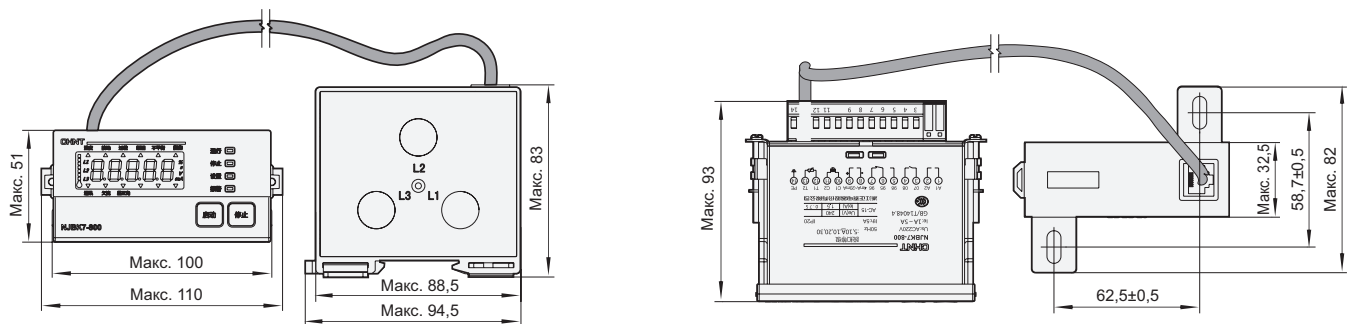
Рис. 2. Габаритные и установочные размеры устройства защиты с номинальным током 5, 10, 40 А
