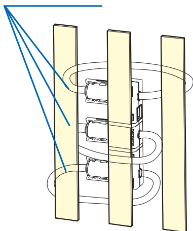
Рис. 5. Вариант 1 установки трансформатора с поясом Роговского
