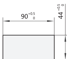
Рис. 7. Размеры монтажного отверстия для блока управления
