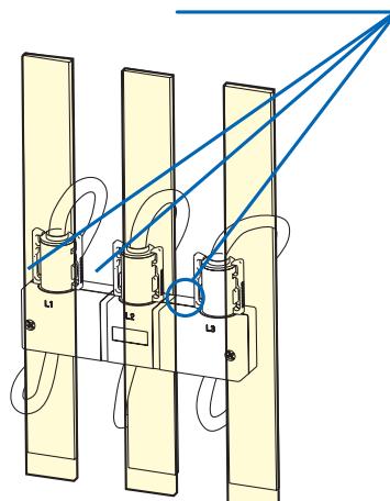
Рис. 6. Вариант 2 установки трансформатора с поясом Роговского
