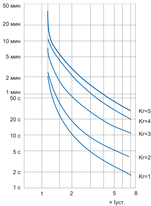
Рис. 1. Время-токовая характеристика
