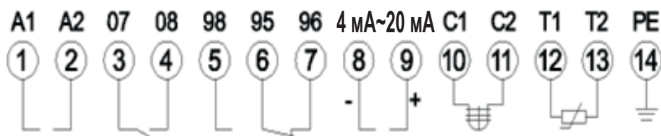
Рис. 9. Обозначения контактов
