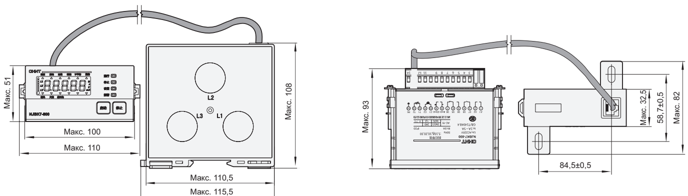
Рис. 3. Габаритные и установочные размеры устройства защиты с номинальным током 100 А
