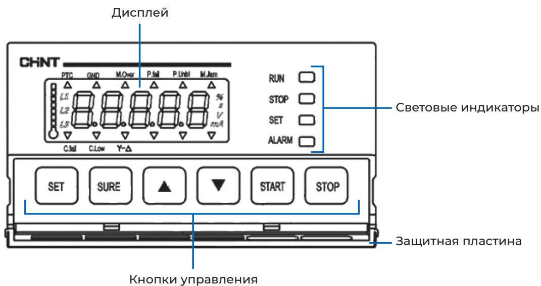
Рис. 8. Схема панели
