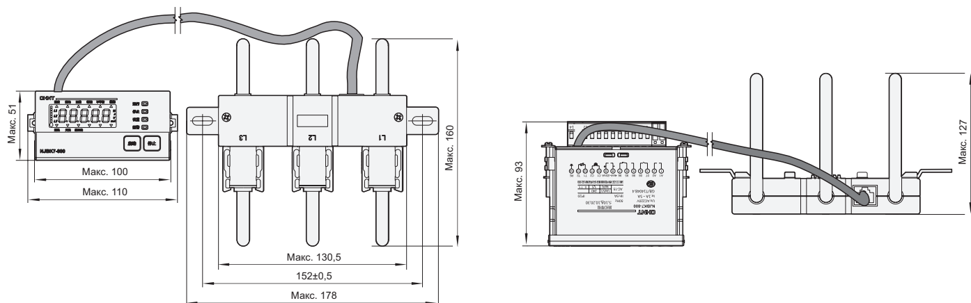
Рис. 4. Габаритные и установочные размеры устройства защиты с номинальным током 400, 800 А
